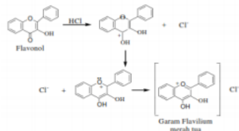
Gambar 4. mekanisme reaksi
